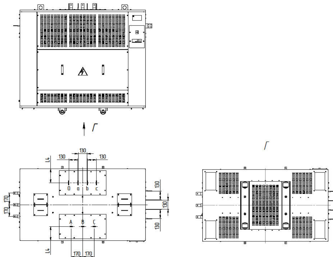
Рисунок Ж.3 – Присоединительные размеры трансформаторов серии ТЛСЗ (при вводах шин ВН или НН сверху)*
