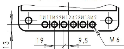
Вторичные выводы М6 с тремя обмотками
