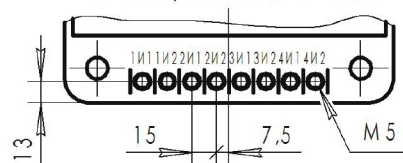
Вторичные выводы М5 с четырьмя обмотками
