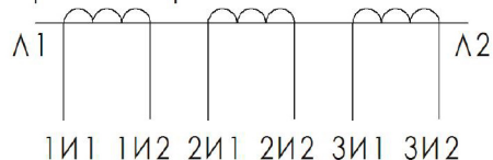
с тремя вторичными обмотками
