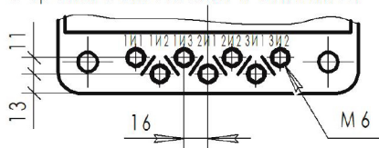
Вторичные выводы М6 с тремя обмотками и отпайкой
