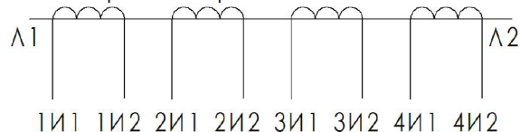
с четырьмя вторичными обмотками
