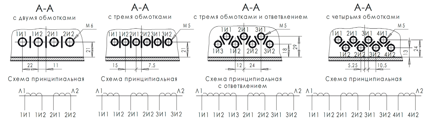
Рисунок 1. Расположение вторичных выводов трансформаторов ТЛК-СТ-10-3, 4, 4М, 4М1, 9М1, 11, 13 на металлическом основании
