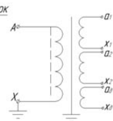
Рисунок Б.4 Принципиальная электрическая схема трансформатора ЗНОЛ06.4-35
