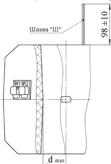
Рисунок Б.2 Общий вид трансформаторов тока ТШЛ-10-1, ТШЛП-10-1. Остальное см. рисунок Б.1
