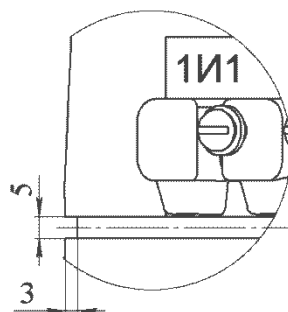
Рисунок Б.3 Общий вид трансформаторов тока ТШЛПК-10, ТШЛК-10, остальное см. рисунок Б.1 и ТШЛПК-10-1, ТШЛК-10-1, остальное см. рисунок Б.2
