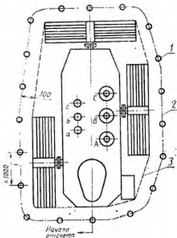
1 — микрофон; 2 — измерительная линия; 3 — излучающая поверхность
