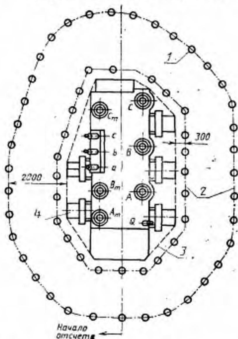
1 — микрофон; 2 — измерительная линия; 3 — излучающая поверхность; 4 — охладитель
