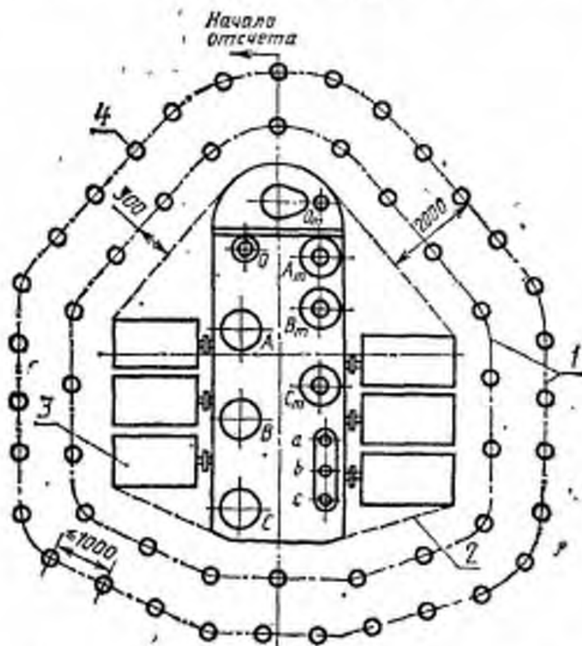
1 — измерительная линия; 2 — излучающая поверхность; 3 — охладители; 4 — микрофон
