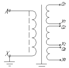
Рисунок А.3 Принципиальная электрическая схема для исполнений ЗНО/106.4
