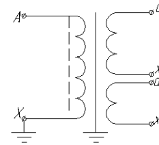
Рисунок А.2 Принципиальная электрическая схема трансформаторов ЗНО/106
