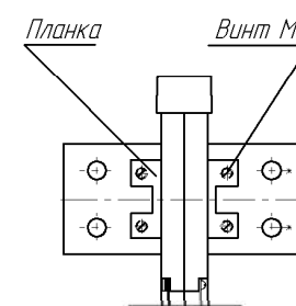
Рисунок А.7 - Крепление шины в окне трансформатора ТШП-0,66
