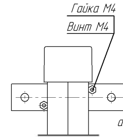
Рисунок А.7 - Крепление шины в окне трансформатора ТШП-0,66
