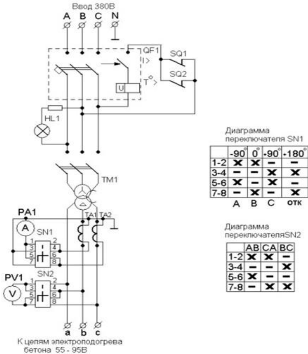
Схема электрическая принципиальная КТПТО - 80
